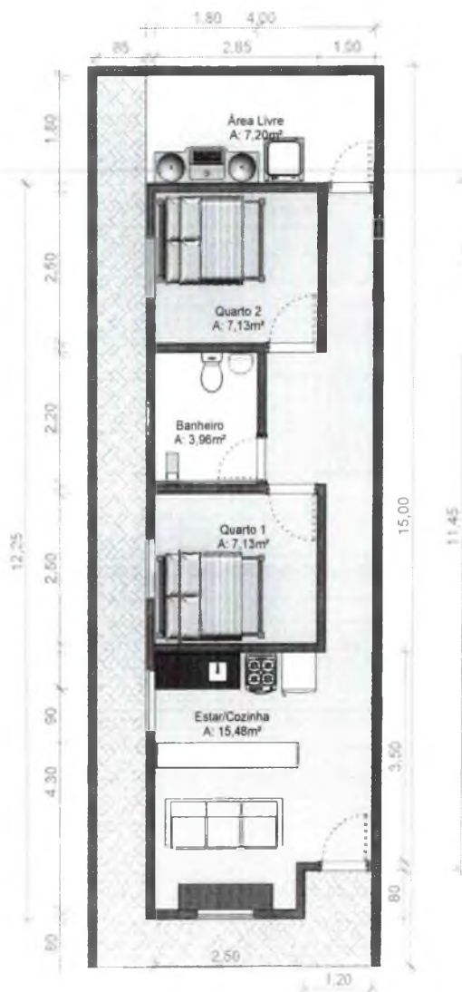
1 PLANTA BAIXA 1 : 75
